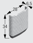
Abdeckung zu Tragwinkel
