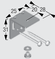
Tragwinkel 28 mm, inkl. Schrauben
