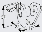
Sicherheitshalterung
