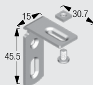
Winkel zu Montageprofil
