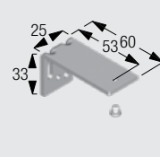
Tragwinkel 60 mm, inkl. Schrauben
