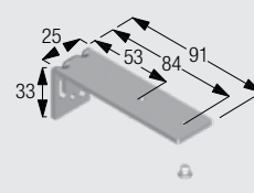
Tragwinkel 91 mm, inkl. Schrauben
