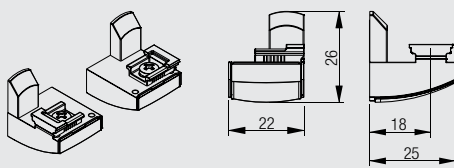
Glasleistenträger inkl. Schrauben
